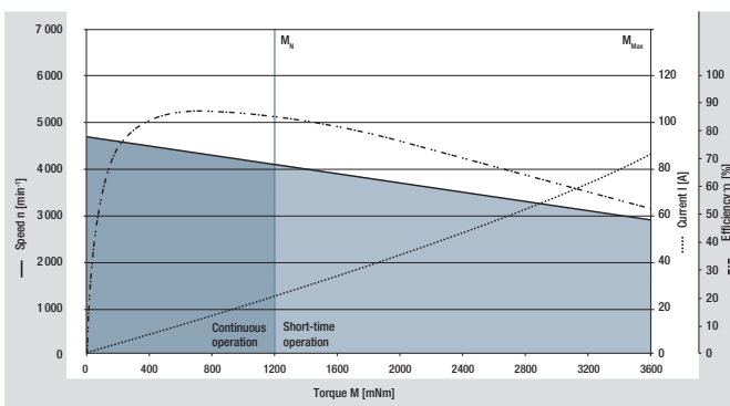
B ECI-80.40-K1, 24 V (at 25 °C)
