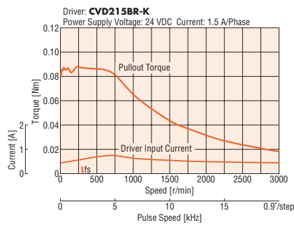
PKP223MD15A/PKP223MD15B
