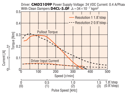
PKP244U04A/PKP244U04B
