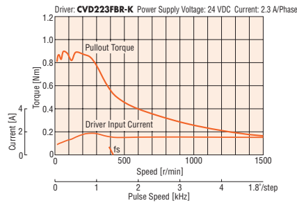
PKP246D23M2
